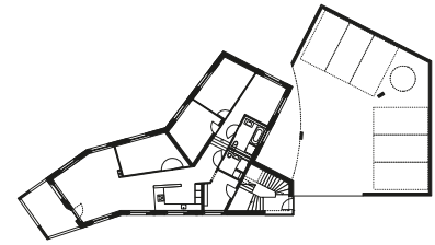
GRUNDRISS EBENE 1
