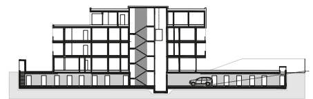
SCHNITT
