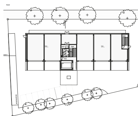
GRUNDRISS EG
