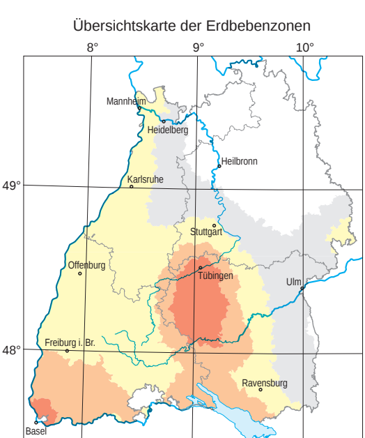
Karte der Erdbebenzonen und geologischen Untergrundklassen für Baden-Württemberg 1: 350 000
